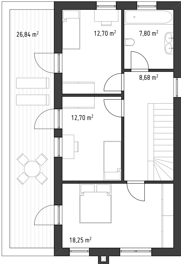
Einfamilienhaus Typ A Grundriss Obergeschoss
